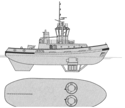
Vue d'un remorqueur
